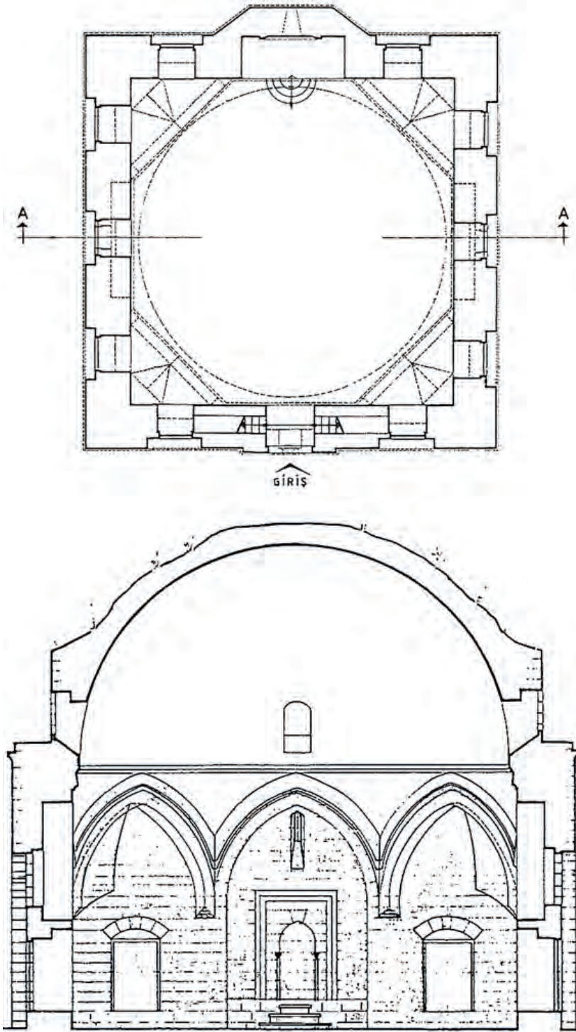
Belge 9) 1973 yılında Semâhâne Cami'ye dönüştürülürken çizilen Cami'nin planı ve kesiti (Vakıflar Genel Müdürlüğü Arşivi)
